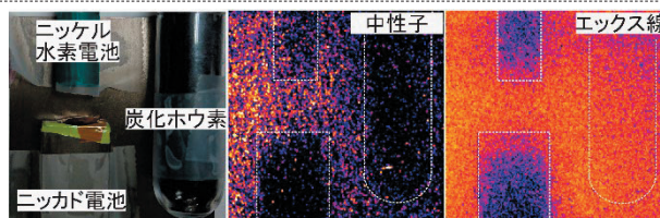
図1:レーザー中性子・X線同時撮像。中性子の透過率からニッケド電池内部のカドミウムの厚さを評価した。
