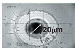
355nmレーザー(LBO) ボロシリケートガラスへのマイクロピア加工(三菱電機資料)
