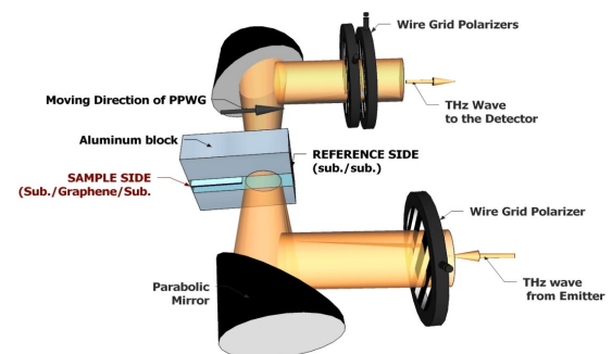
図 平行平板導波路型テラヘルツ分光システムの模式図
