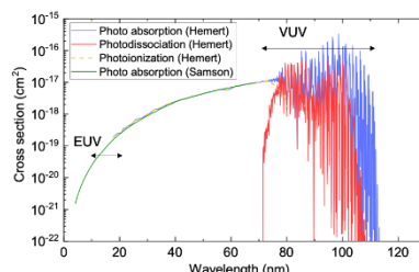
Fig. 2 水素ラジカル生成断面積。光解離過程の方が光電離よりも2桁ほど断面積が大きい。
