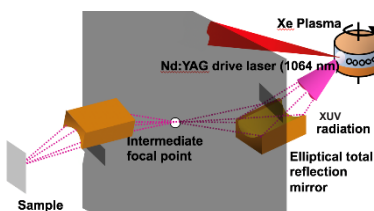
Fig. 2 レーザープラズマXUV光源と集光系。 N. Tanaka et al, HEDP 37, 100865 (2020)他
