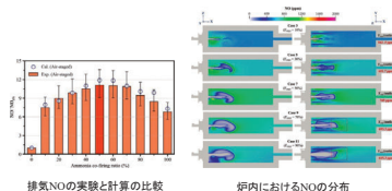
排気NOの実験と計算の比較
