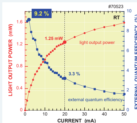
Eu 添加 GaN 赤色 LED の特性
