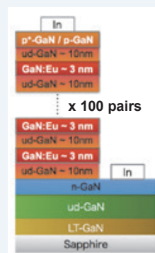
Eu 添加赤色 LED の構造
