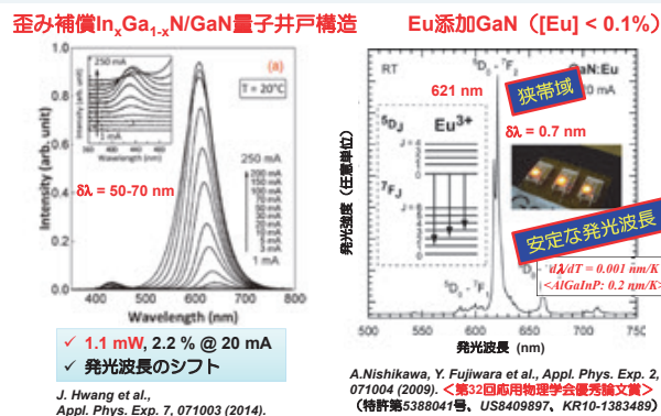
従来の赤色 LED (InGaInP) と今回の赤色 LED (EuGaInP) の比較
